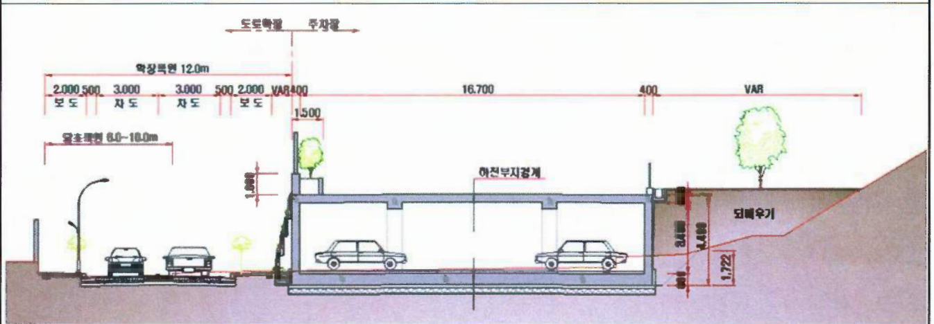
단면도(안)
