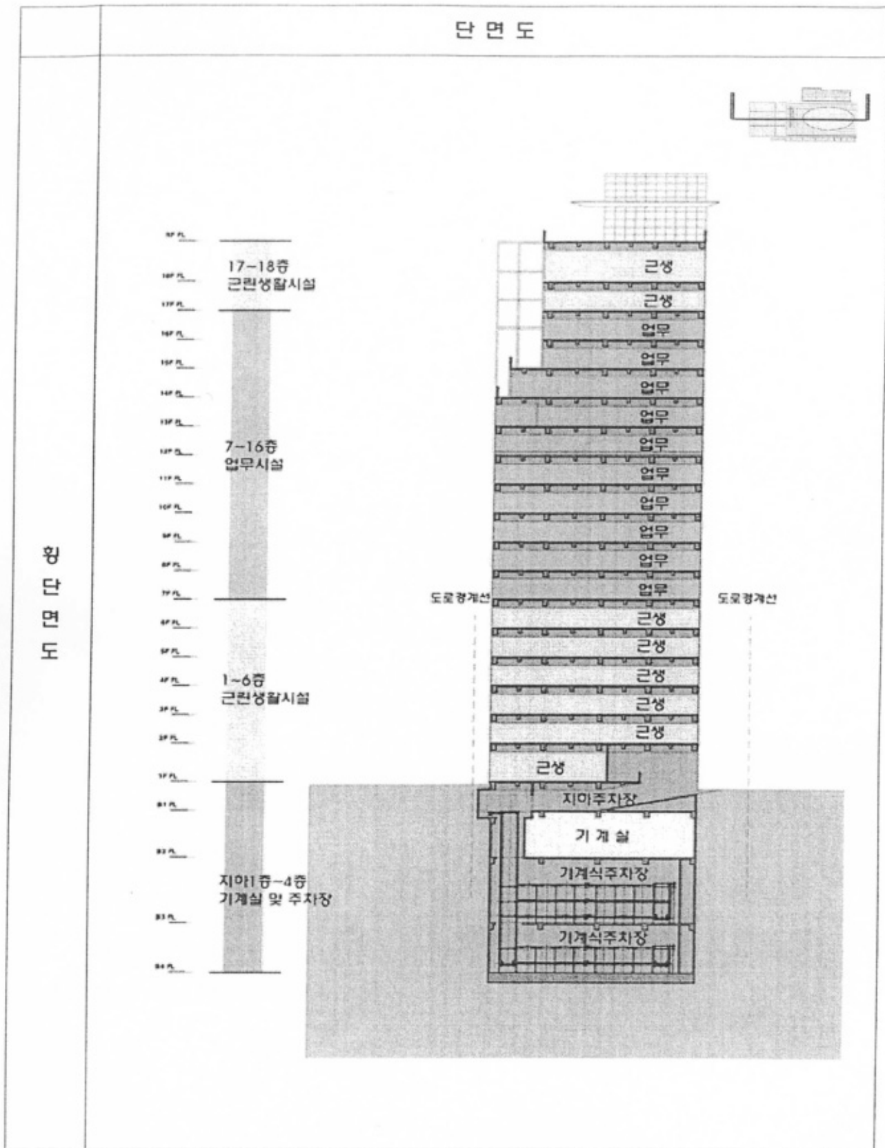
라. 단면도
